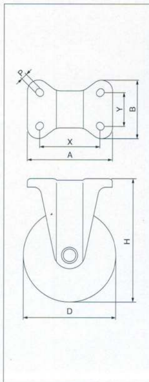
平付けプレートタイプ 固定
