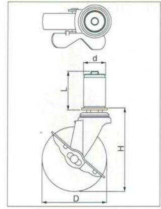
ETF-S 自在ストッパー型
