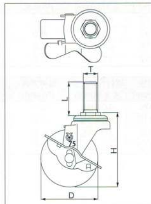
SUS-ST-S 自在ネジ込ストッパー型
