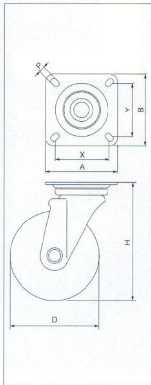
平付けプレートタイプ 自在
