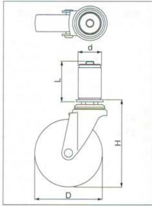
ETF-S 自在ストッパー型
