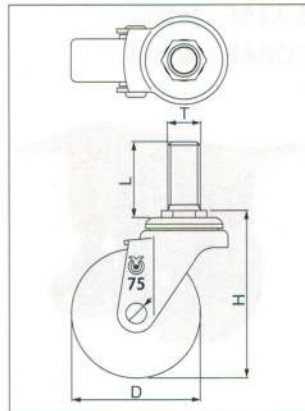
SUS-ST 自在ネジ込型
