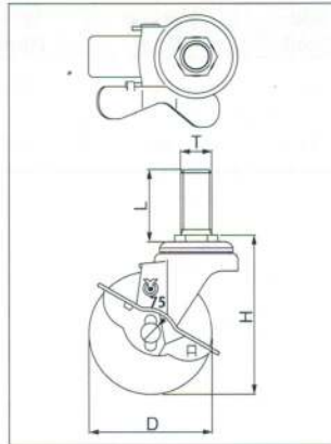
ST-S 自在ネジ込ストッパー型
